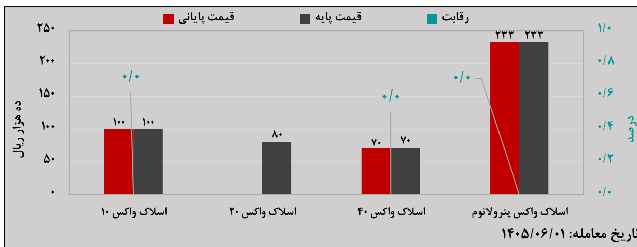
شکل ۱۰. میزان رقابت قیمتی انواع اسلاک واکس شرکت نفت ایرانول تهران؛ هفته اول شهریور ۱۴۰۵
